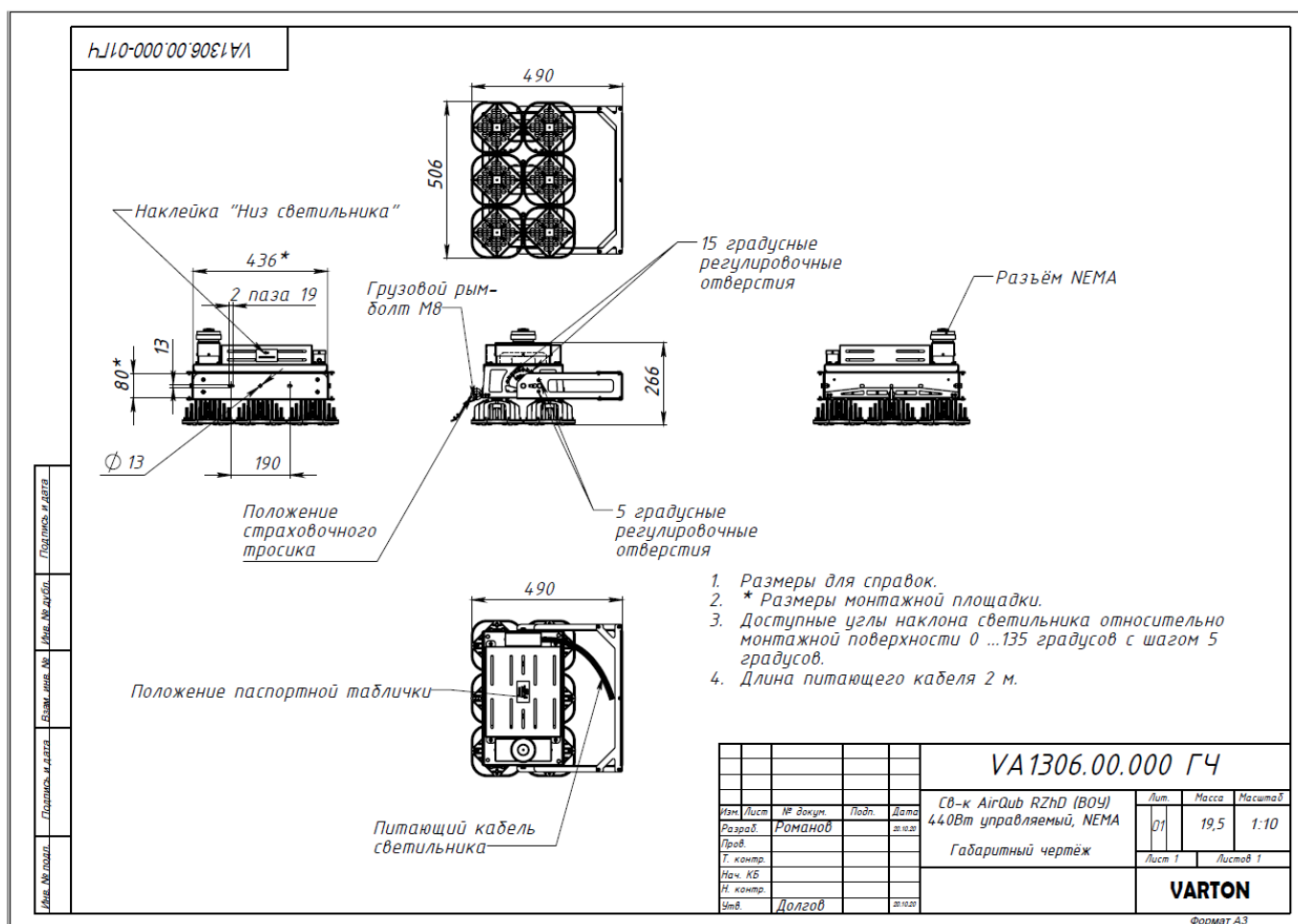
Габаритный чертёж светильников VA1306.00.000 AirQub RZhD 440 Вт
